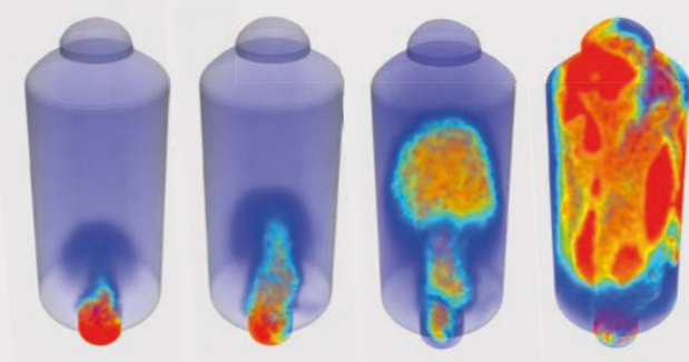
горение водородосодержащей смеси в замкнутом объеме
