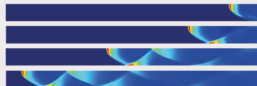
распространение горения в стратифицированной водородосодержащей смеси
