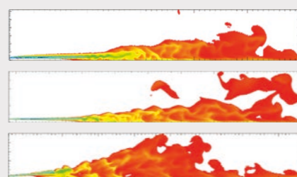
моделирование гильотинных разрывов трубопроводов с горючими газами при риформинге природного газа
